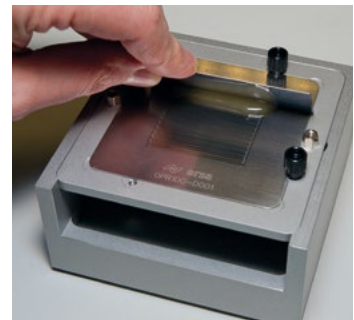
Flussmittelauftrag in Dip-Schablone
