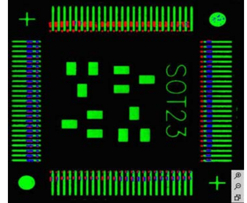
Computerunterstützte Ausrichtung eines OFP grün: Landflächen, rot: Bauteilanschlüsse, blau: optimale Überlagerung
