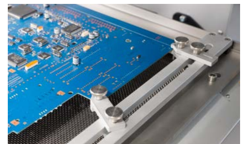
Flexible Leiterplattenhalterung
